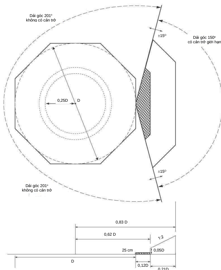
Hình 7 - Dải góc có cản trở giới hạn của sân bay: máy bay trực thăng một cánh quạt chính
