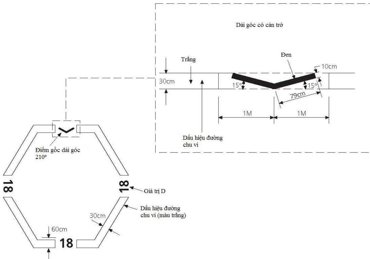
Hình 8 - Dấu hiệu dải góc không có cản trở
